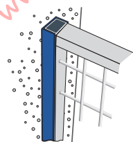
Wandverbindung aus U-Profil 32 x 30 x 1,5 mm
