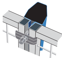
Zwischenständer mit 2 montierten Wandelementen
