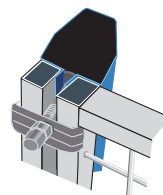
Endständer mit 1 Wandelement und Vierkantrohr als Abschluss
